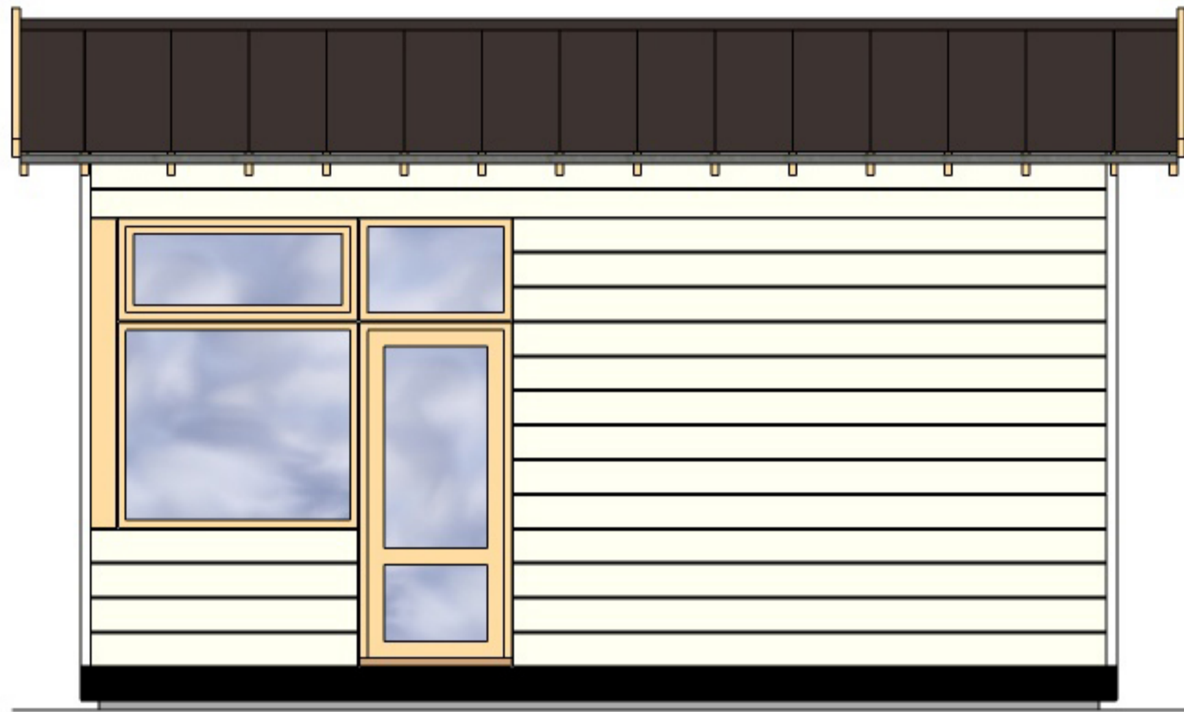
LÅNGSIDA
